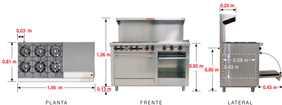
PLANTA
